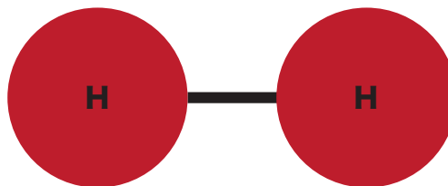
水素分子
