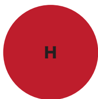
水素原子
