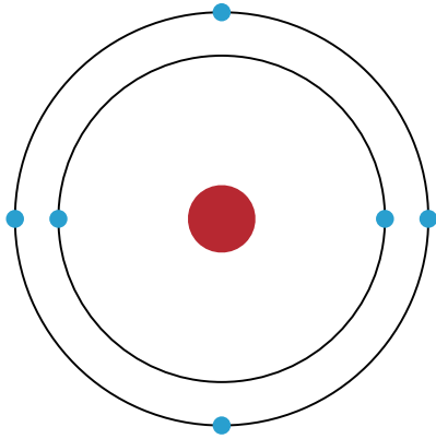
例) 炭素 C (原子番号 6)
